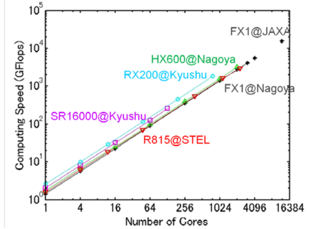
Fig. 6 ブラソフコードの弱いスケールリング (40x20x30x30x30/core)。
