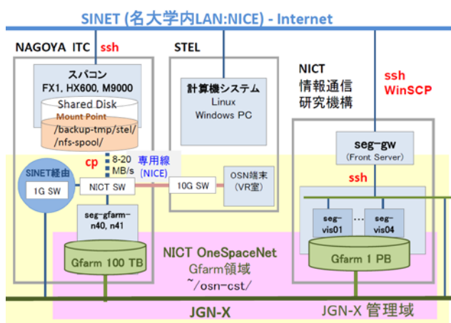
Fig.11 JGN-X で構築された広域分散ファイルシステム (Gfarm) と NICT OneSpaceNet を用いた地球磁気圏 3 次元 MHD シミュレーションの画像処理。
