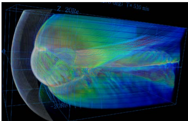
Fig. 2 地球のダイポール固有磁場に傾きがある場合の地球磁気圏の高精度 3 次元 MHD シミュレーション、磁気圏境界層で渦乱流が形成されている。
