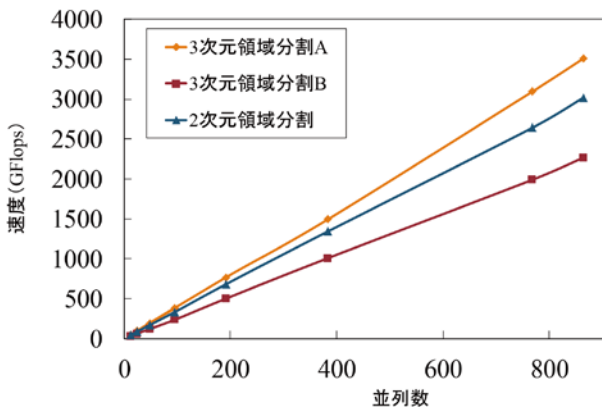
Fig. 1 九州大学新システムにおける性能評価。Intel Xeon X5670 は擬似ベクトル化の効果が発揮されるのでベクトル長と通信量がバランスした 3 次元領域分割方が高効率である。
