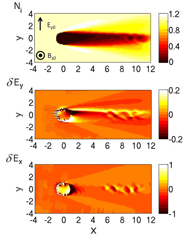
Fig.7 イオン密度及び電場 E_x と E_y 成分。左側境界より太陽風粒子及び惑星間磁場(IMF: B_z 成分)が流入。
