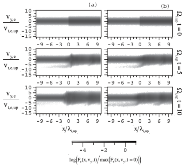
Fig. 5 電子の x - v_x 位相密度。(a) y 方向の空間領域がイオン慣性長の 5 倍。(b) y 方向の空間領域がイオン慣性長の 1 倍
