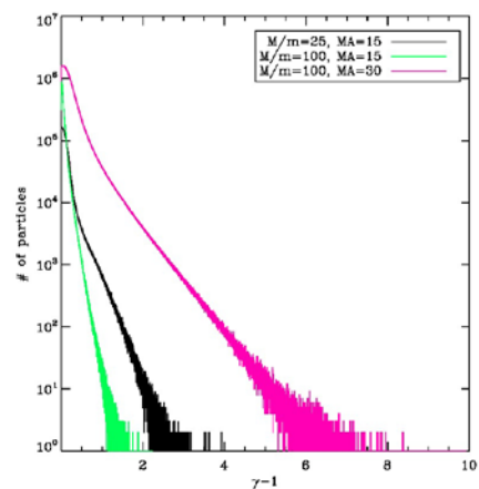
Fig. 3 衝撃波下流での電子のエネルギースペクトル
