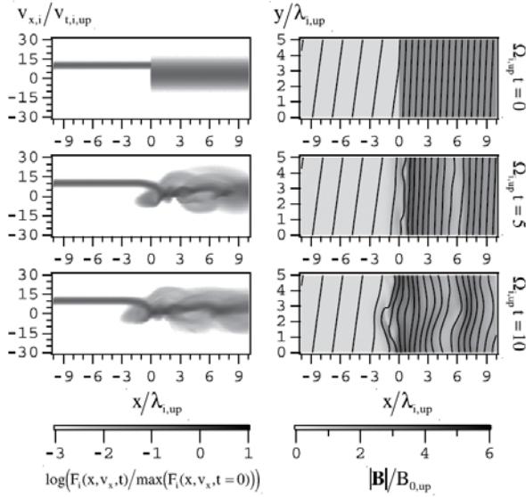
Fig. 4 (左)イオンの x - v_x 位相密度及び(右)磁場成分 B_y の強度と磁力線
