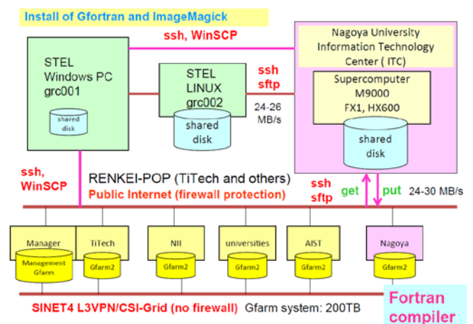
Fig.10 RENKEI-PoP プロジェクトで構築された広域分散ファイルシステム (Gfarm) を用いた地球磁気圏 3 次元 MHD シミュレーションの画像処理。
