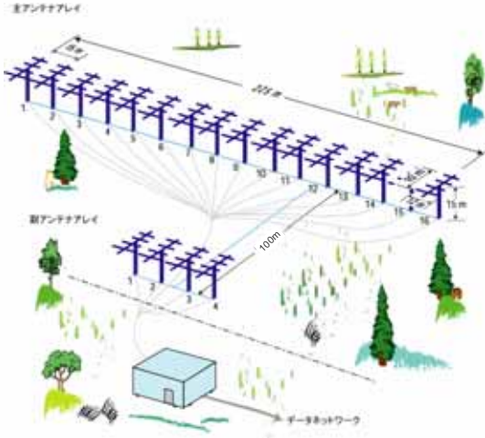
レーダーアンテナ・送受信装置の概観図
