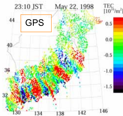
日本国内観測網 (共同研究実施中)
